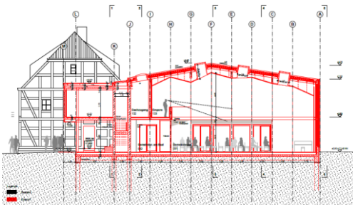
Planungsskizze des Neubaus unseres Tobias-Seiler-Saales
